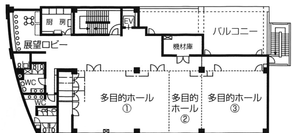
<2階平面図>
